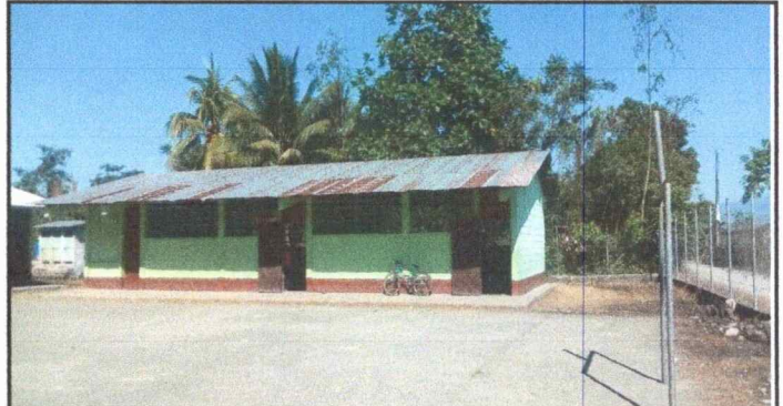
Foto 2: Se observa el deterioro de las laminas portantes del modulo 2
